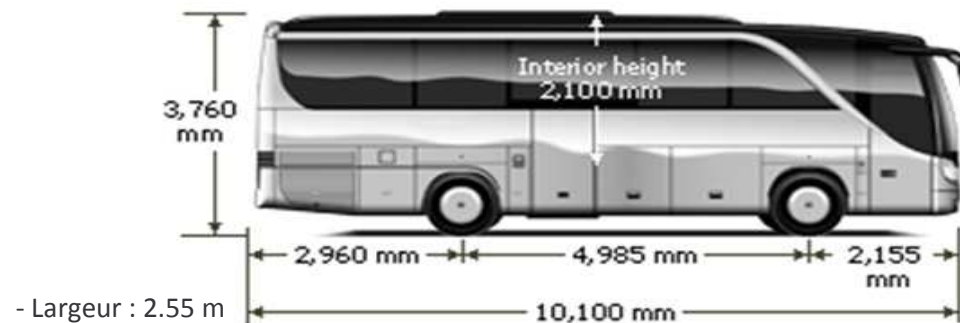
MESURES EXTERIEURES
